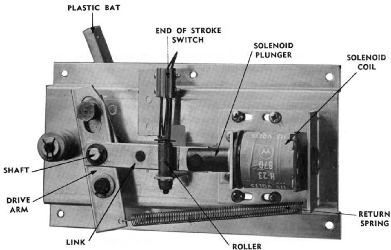
BATTER UNIT
